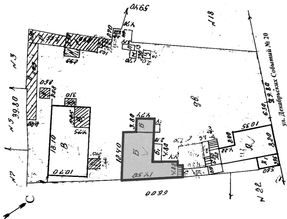
Рис. 2 - Схема генплана по материалам БТИ за 1979 год.
