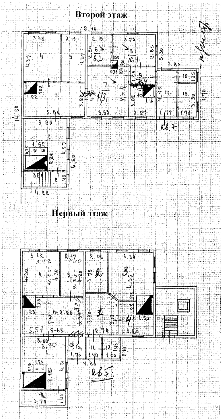
Рис. 3 - поэтажные планы БТИ за 1985 год.
