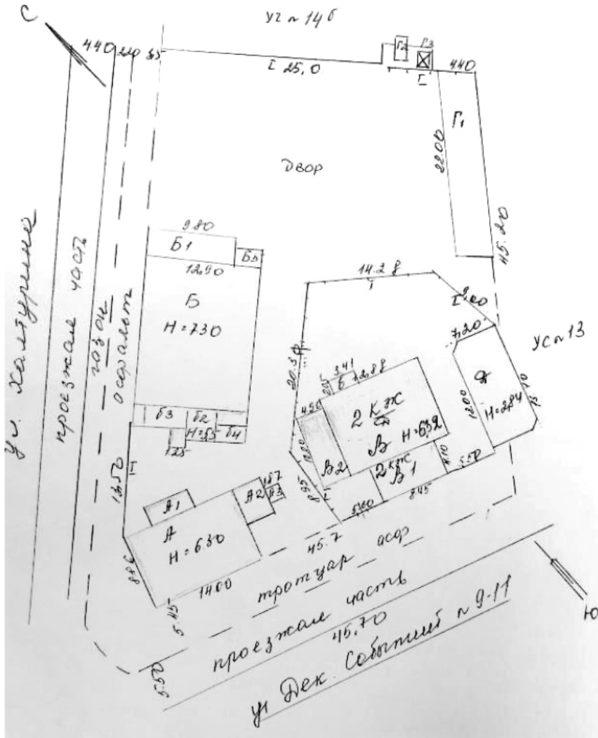
Рис. 1 - Генплан участка по ул. Декабрьских Событий, 9
