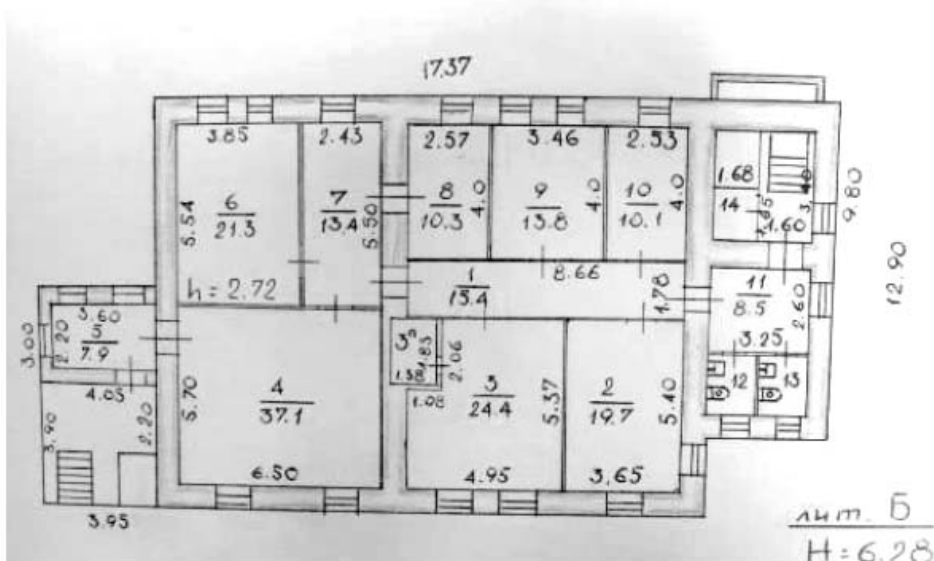
Рис.2 - поэтажные планы доходного дома по ул. Декабрьских Событий, 9 (лит. Б) (инвентаризация БТИ 2006 г.)
