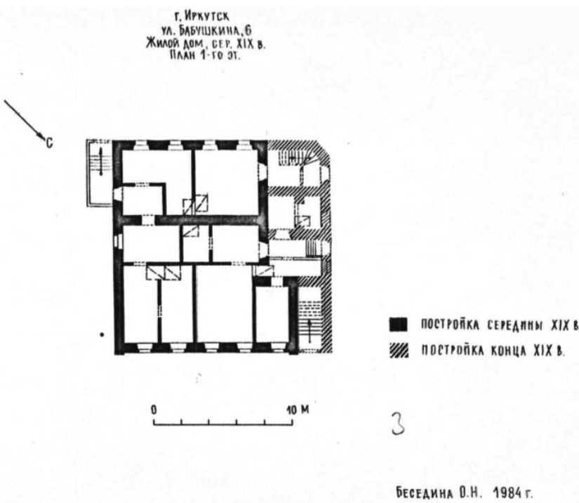
Рис. 2. План 1-го этажа. Чертеж Бесединой О.Н. Паспорт объекта культурного наследия – 25.01.1984 г.
