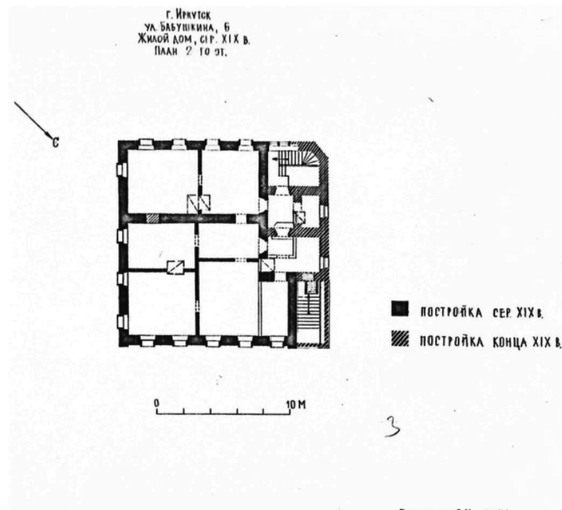
Рис. 3. План 2-го этажа. Чертеж Бесединой О.Н. 1984 г. Паспорт объекта культурного наследия – 25.01.1984 г.
