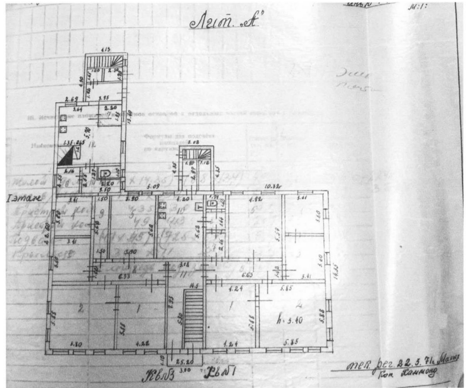
Рис. 4. План БТИ
