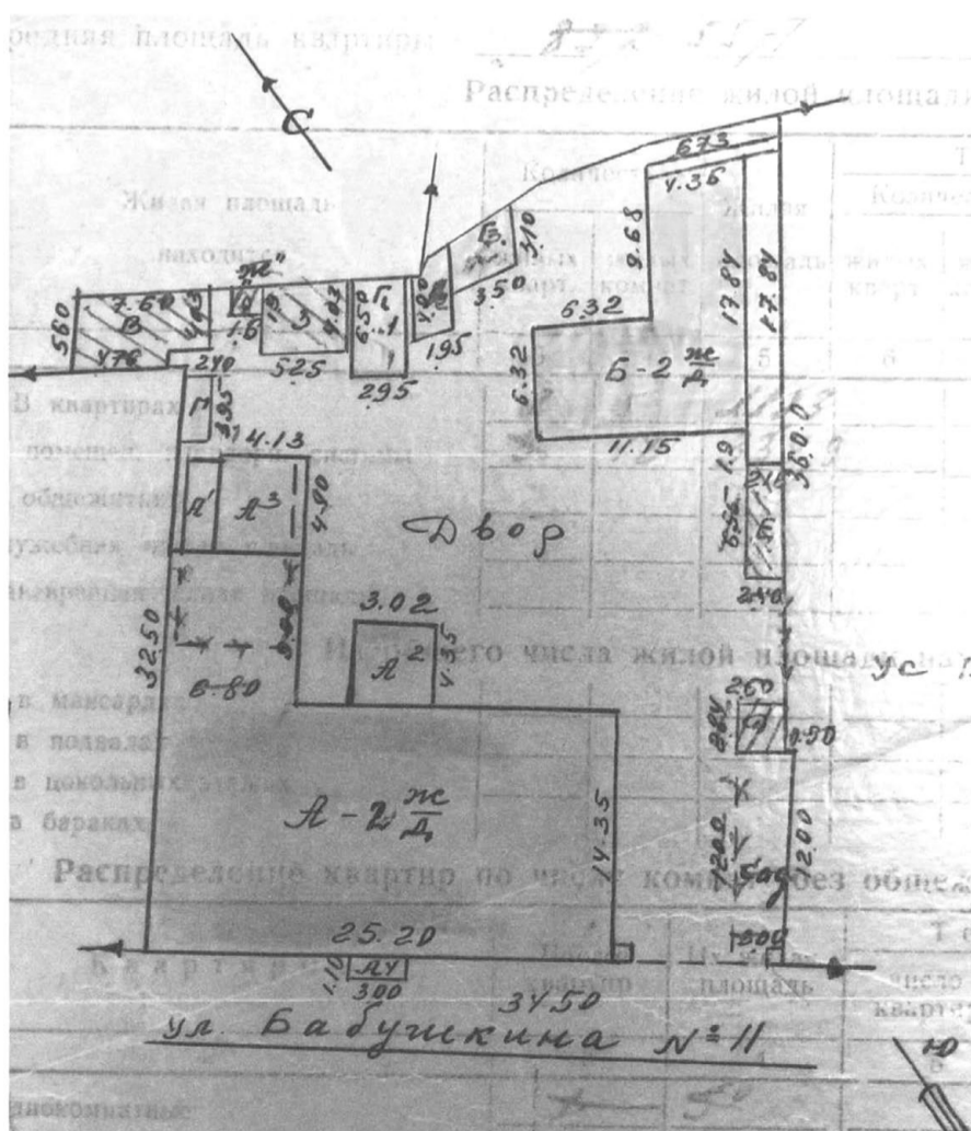
Рис. 3. План БТИ
