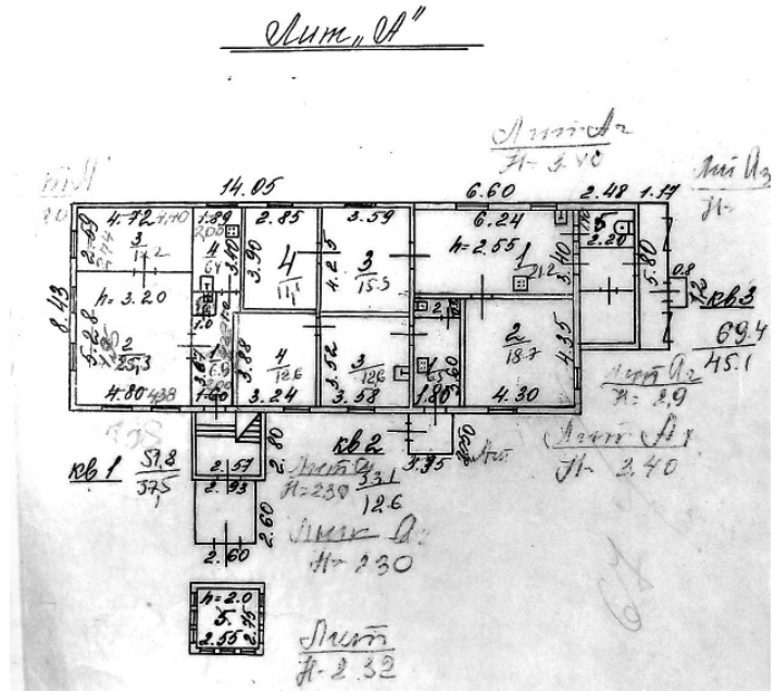
Рис. 2 - поэтажный план БТИ
