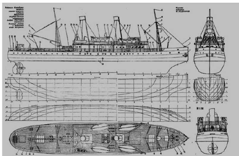
ПРИЛОЖЕНИЕ 1. Подлинные чертежи проекта ледокола «Ангара». Общий вид судна. Экспонат экспозиции на судне.
