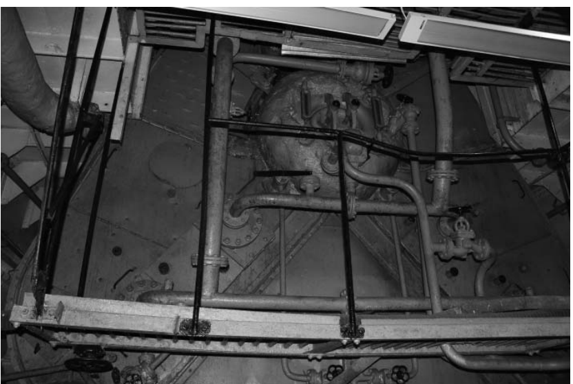
Фото А.А. Жильцов, август 2018 г. Вид на верхний барабан парового котла треугольного типа с заваренными топками.
