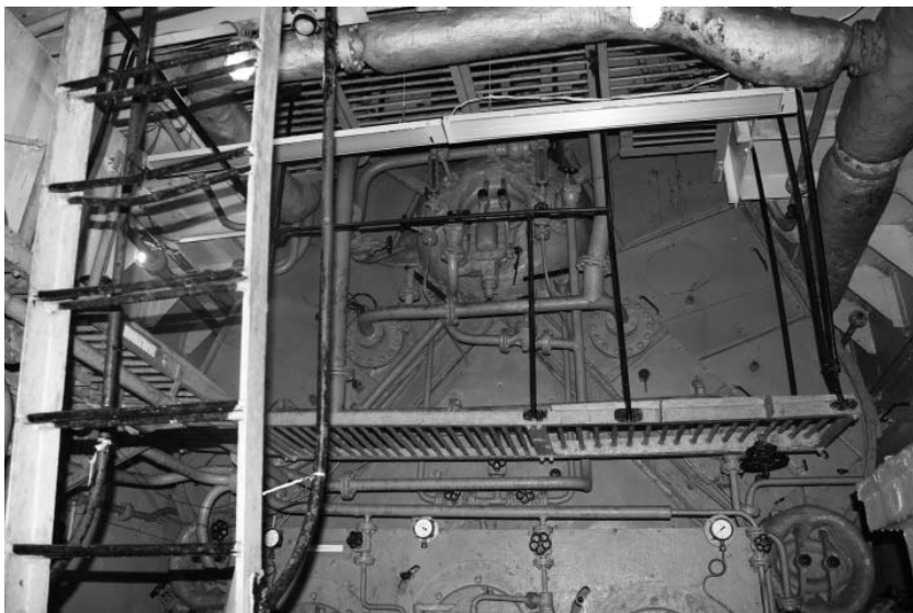
Фото А.А. Жильцов, август 2018 г. Паровой котел треугольного типа с незаваренными топками.
