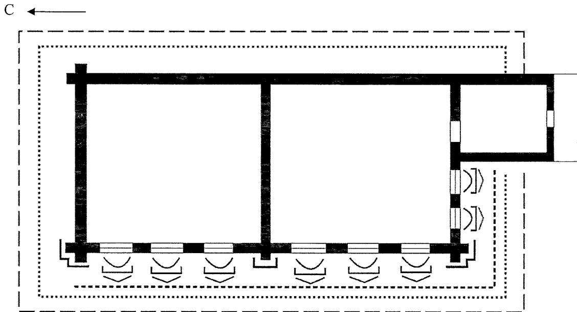
Схема обозначения предмета охраны в уровне первого этажа
