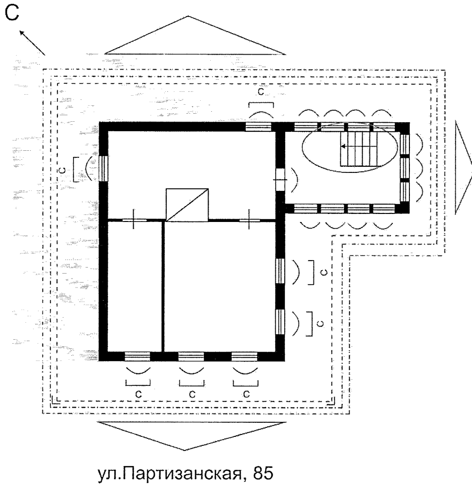
Схема 2 этажа
