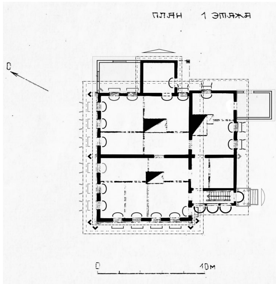
Схема расположения предмета охраны (ценных элементов) 1 этажа
