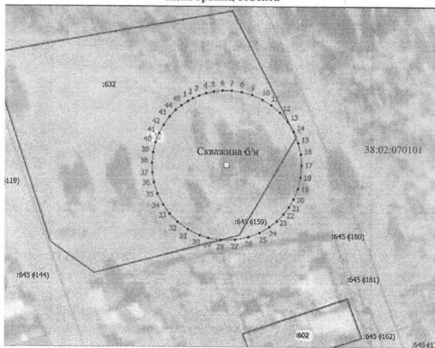
План границ объекта
